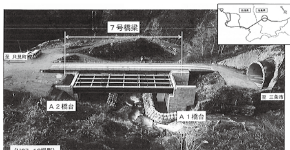
7号橋梁（福島県側）
