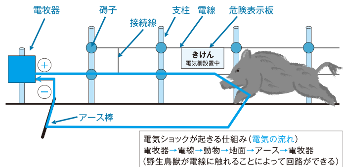
▲電気柵の仕組みの模式図
